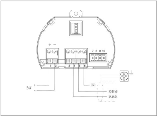
四线制、单腔
